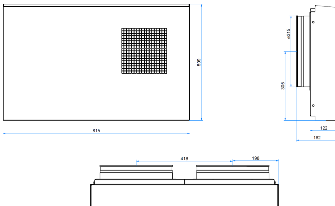
Figur 2: Veggdeksel måltegnning
