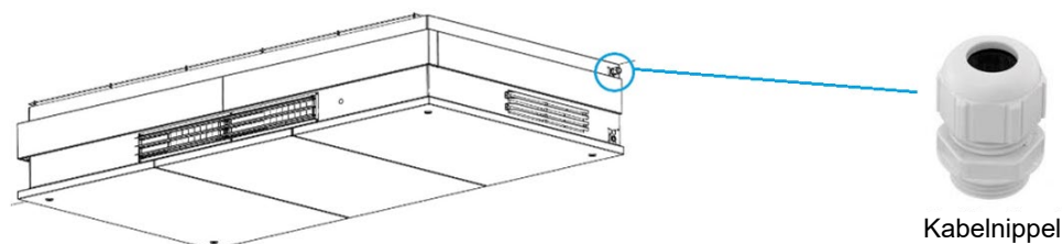
Figur 4: Innføring av forsyningskabel og kabelgjennomføring
