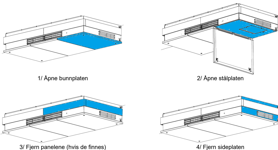
Figur 3: Få tilgang til tilkoblingene
